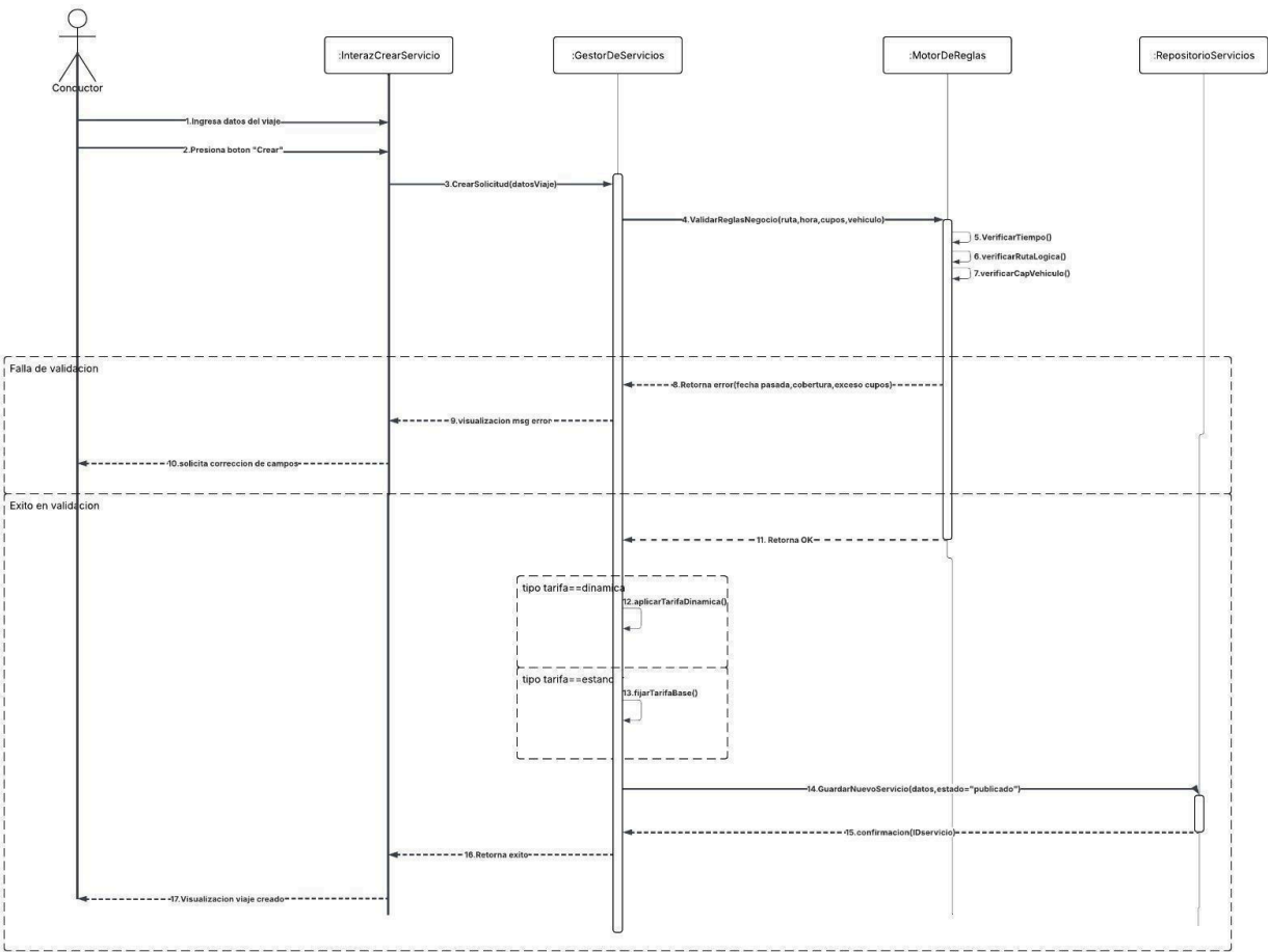
Figura 11. Diagrama de secuencia del módulo Crear viaje.
